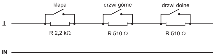
Rys. 4 Schemat połączenia czujników klapy i drzwi.
